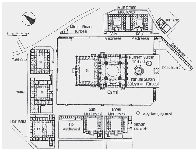
Görsel 10: Süleymaniye Cami ve Külliyesi'nin mimari planı
