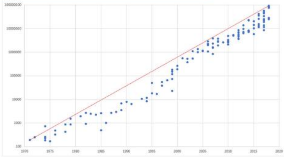
Şekil 9. Bilgisayar mikroişlemcilerinde 1mm 2 ye düşen transistör sayısının yıllara göre değişimi (Kaynak: https://medium.com/predict/moores-law-is-alive-and-well-aaa49a450188 )
